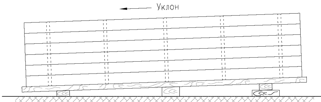
Рис.Хранение транспортного пакета с панелями под открытым небом
